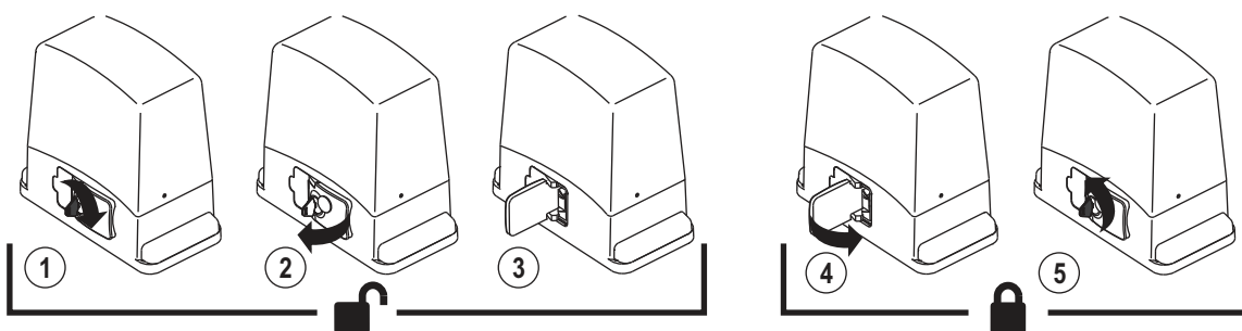
Rysunek 8. Rozsprężanie / zasprężanie napędu bramy
