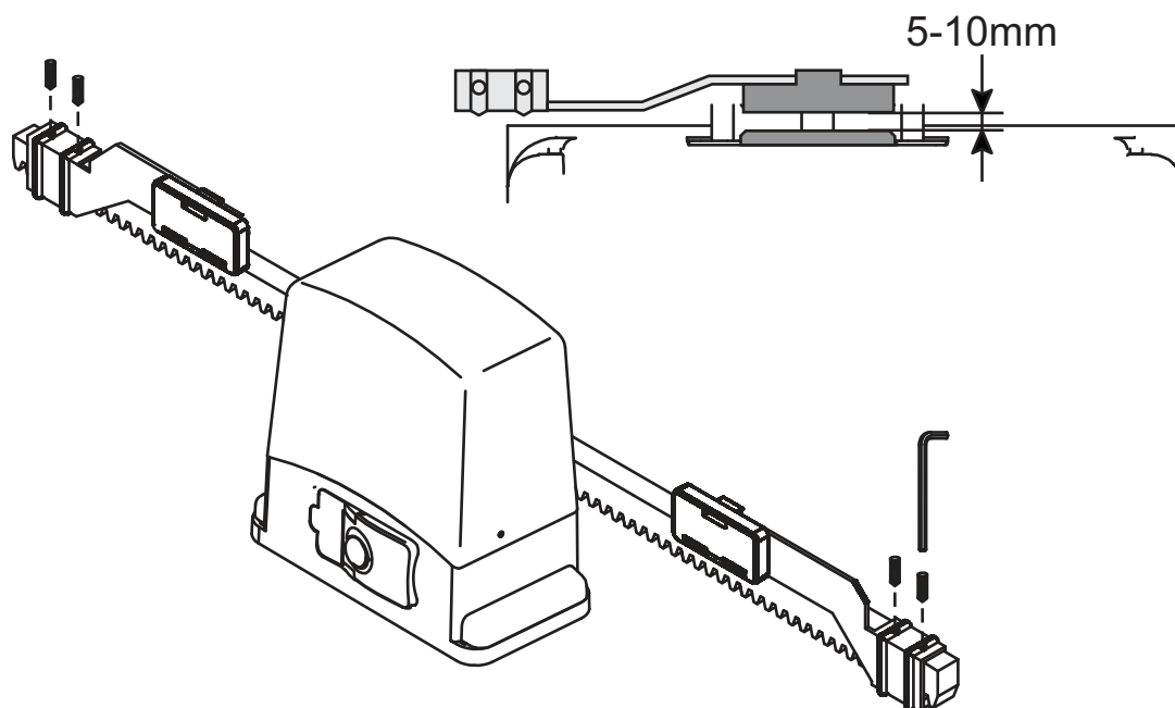
Rysunek 7. Montaż magnesów wyłącznika krańcowego otwierania / zamykania
