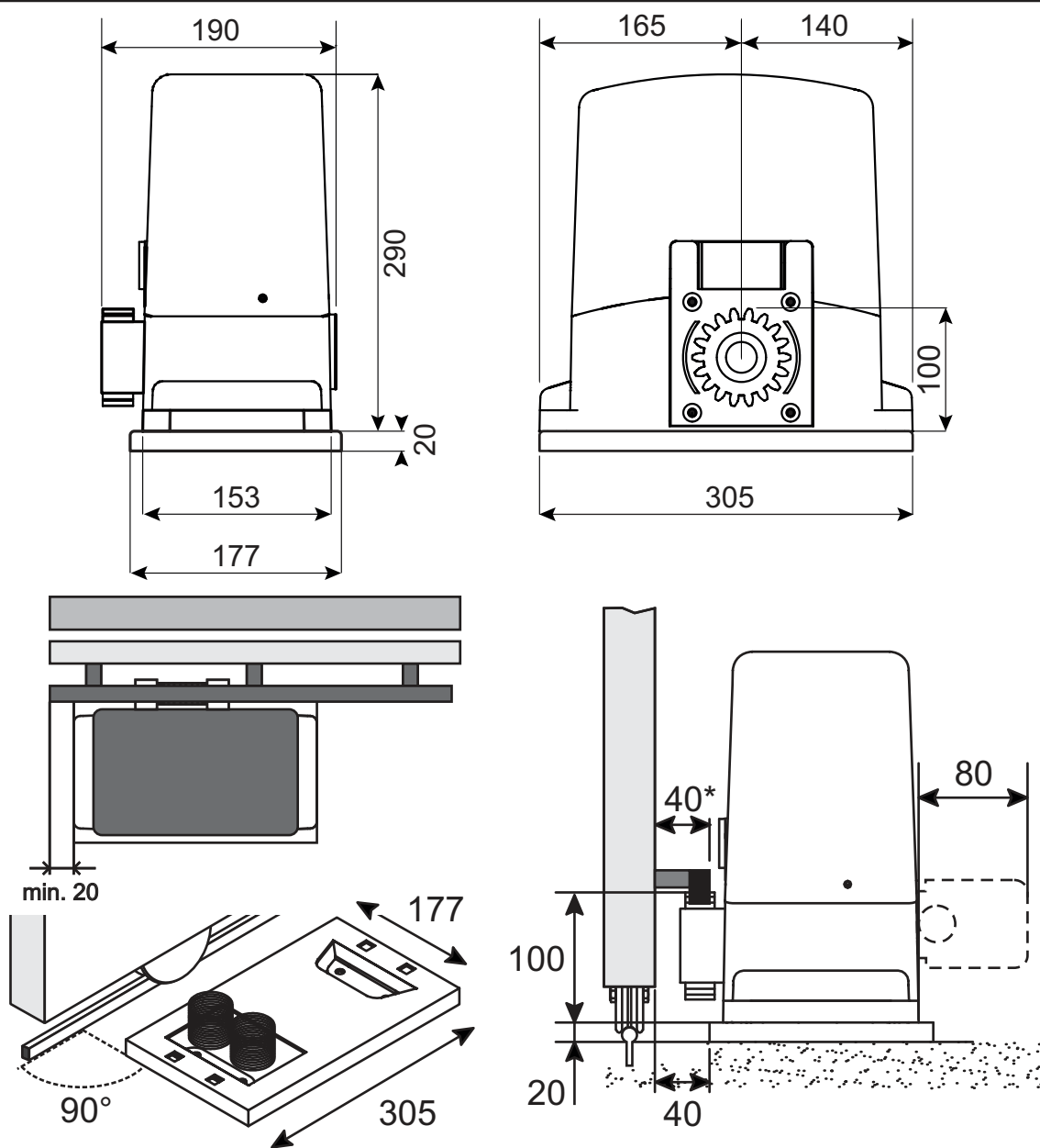
Rysunek 4. Wymiary napędu i zalecane wymiary montażu (mm).
