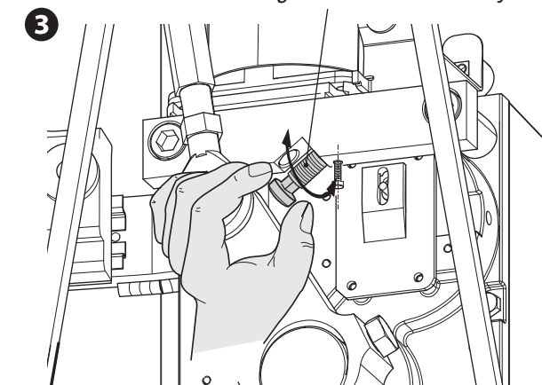
Ogranicznik mechaniczny
