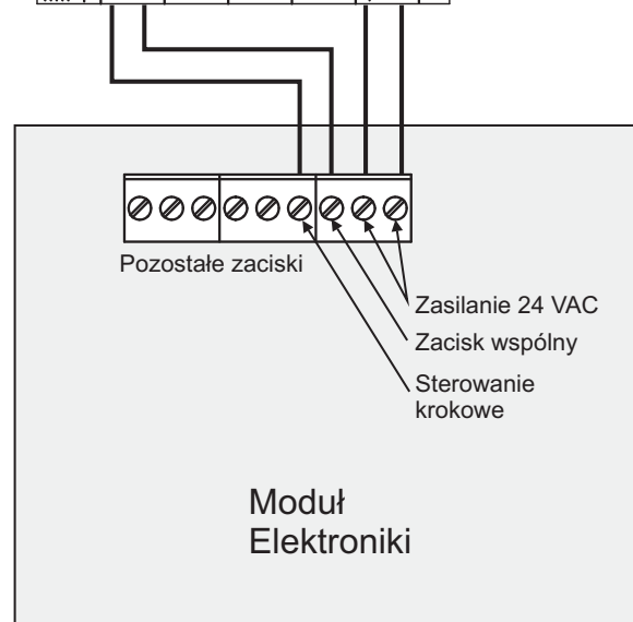
Schemat 4. Przykład połączenia sterownika napędu bramy NICE z odbiornikiem ZSP Rival 434.
