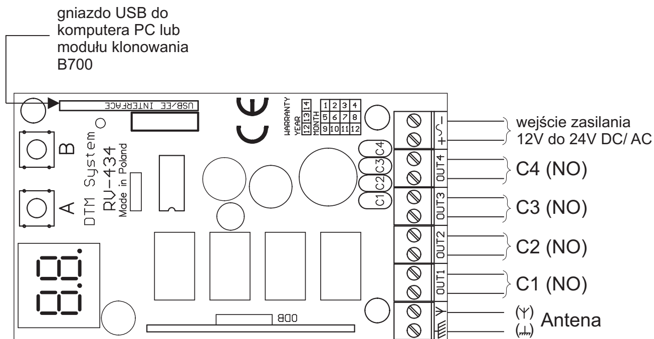
rys 1. Schemat elektryczny instalacji odbiornika Rival 434
