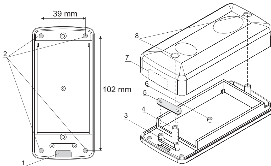
rys.3 Widok obudowy odbiornika Rival 434.
