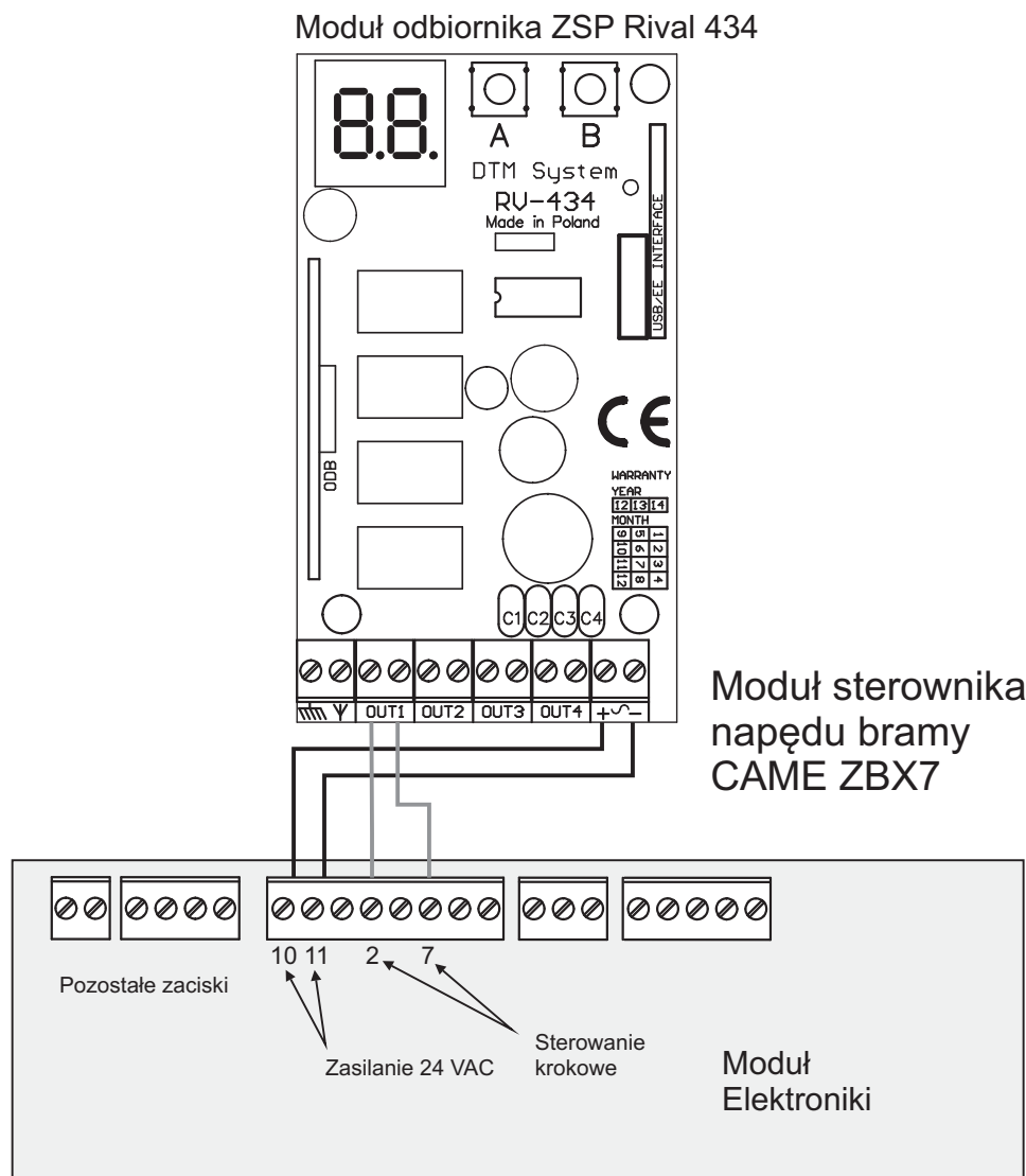
Schemat 1. Przykład połączenia sterownika napędu bramy CAME ZBX7 z odbiornikiem ZSP Rival 434.
