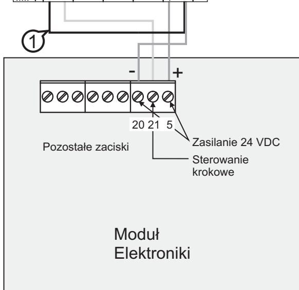
Schemat 3. Przykład połączenia sterownika napędu bramy Hormann z odbiornikiem ZSP Rival 434.
