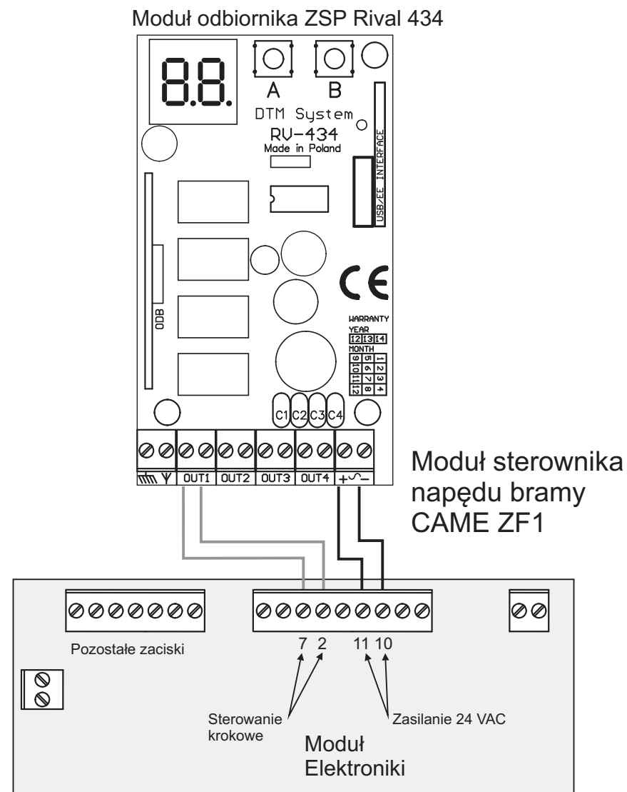
Schemat 2. Przykład połączenia sterownika napędu bramy CAME ZF1 z odbiornikiem ZSP Rival 434.
